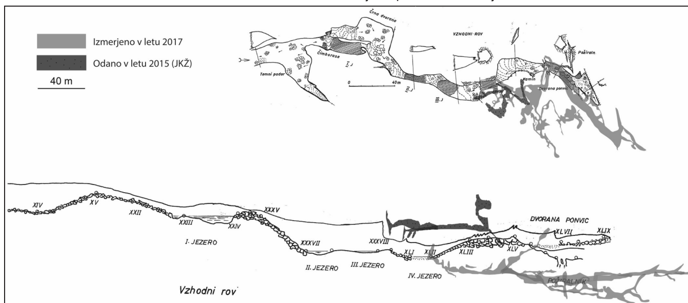
Prikaz lege novo odkritih in raziskanih delov Prepadne jame na originalnem načrtu (načrt prevzet po: D. Novak (1963), Prepadna jama pri Suhorju, kat. št. 2566. Naše jame: 30–36).
