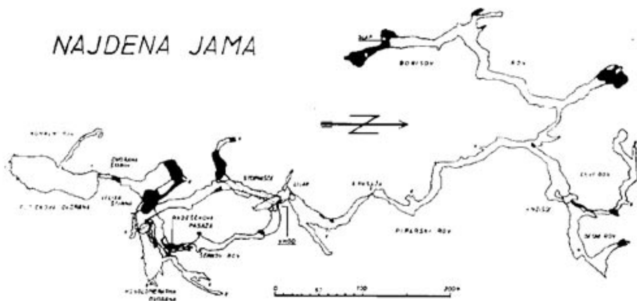
Skica tlorisa Najdene jame, prirejena je po meritvah: S. Pirnata, M. Puca in F. Šušteršiča, ki so jih v celoti opravili s pomočjo mladih članov Jamarskega kluba Ljubljana.
